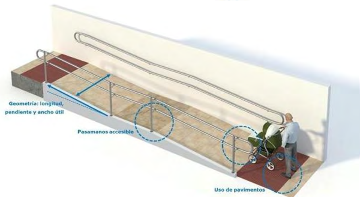
Ilustración 3. Escalera accesible. Fuente: Manual de accesibilidad para espacios públicos urbanizados del Ayuntamiento de Madrid
