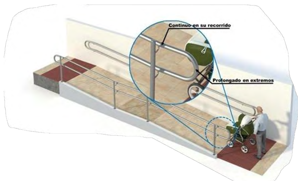
Ilustración 4. Pasamanos accesible. Fuente: Manual de accesibilidad para espacios públicos urbanizados del Ayuntamiento de Madrid
