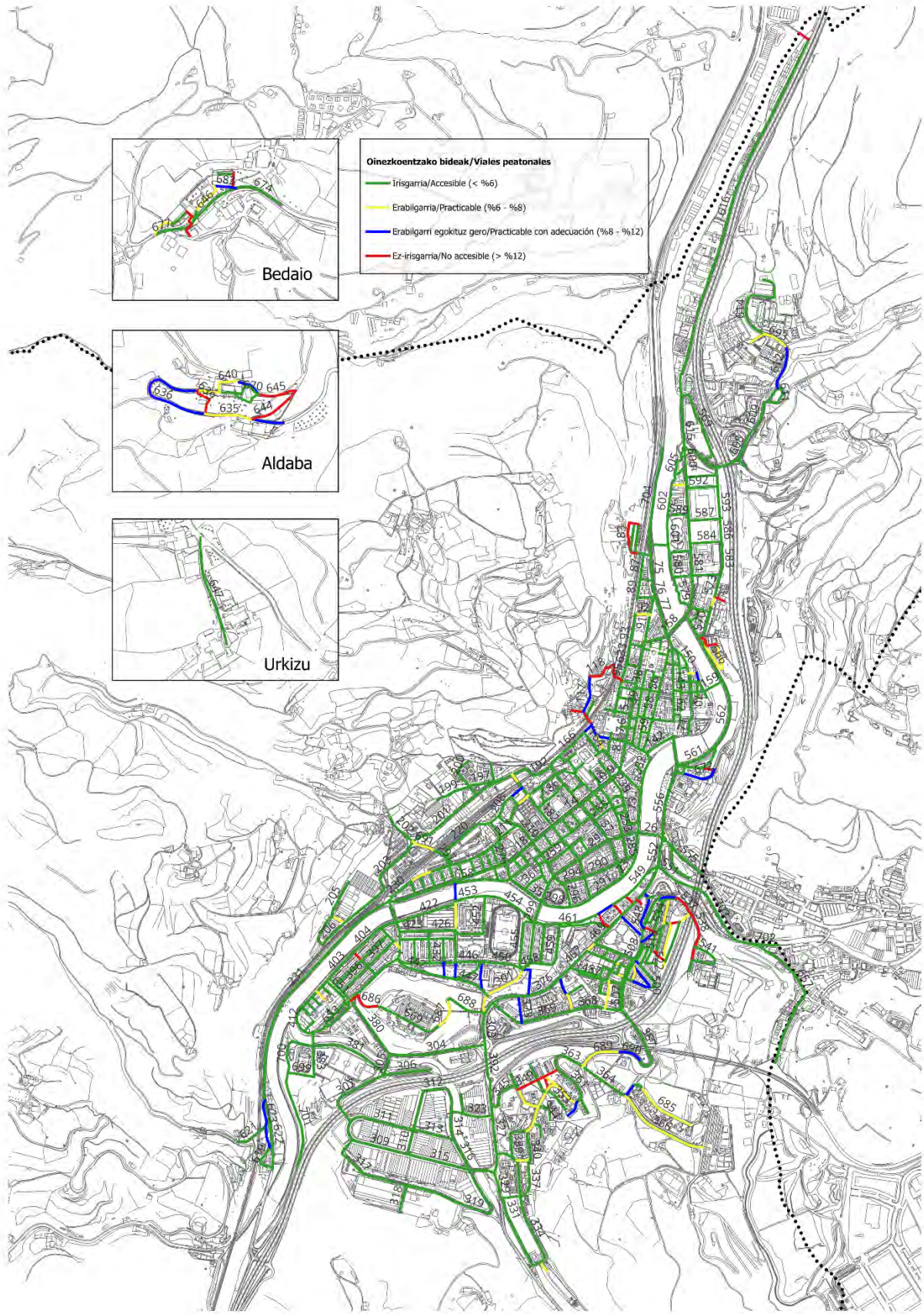
Ilustración 1. Desniveles Vías Peonales
