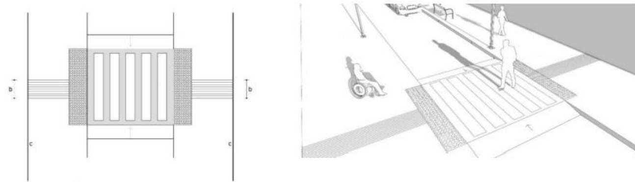
Ilustración 11. Ejemplo Aplicación del pavimento táctil indicar en cruce con paso de peatones elevado. Fuente: Guía de accesibilidad en los espacios públicos urbanizados
