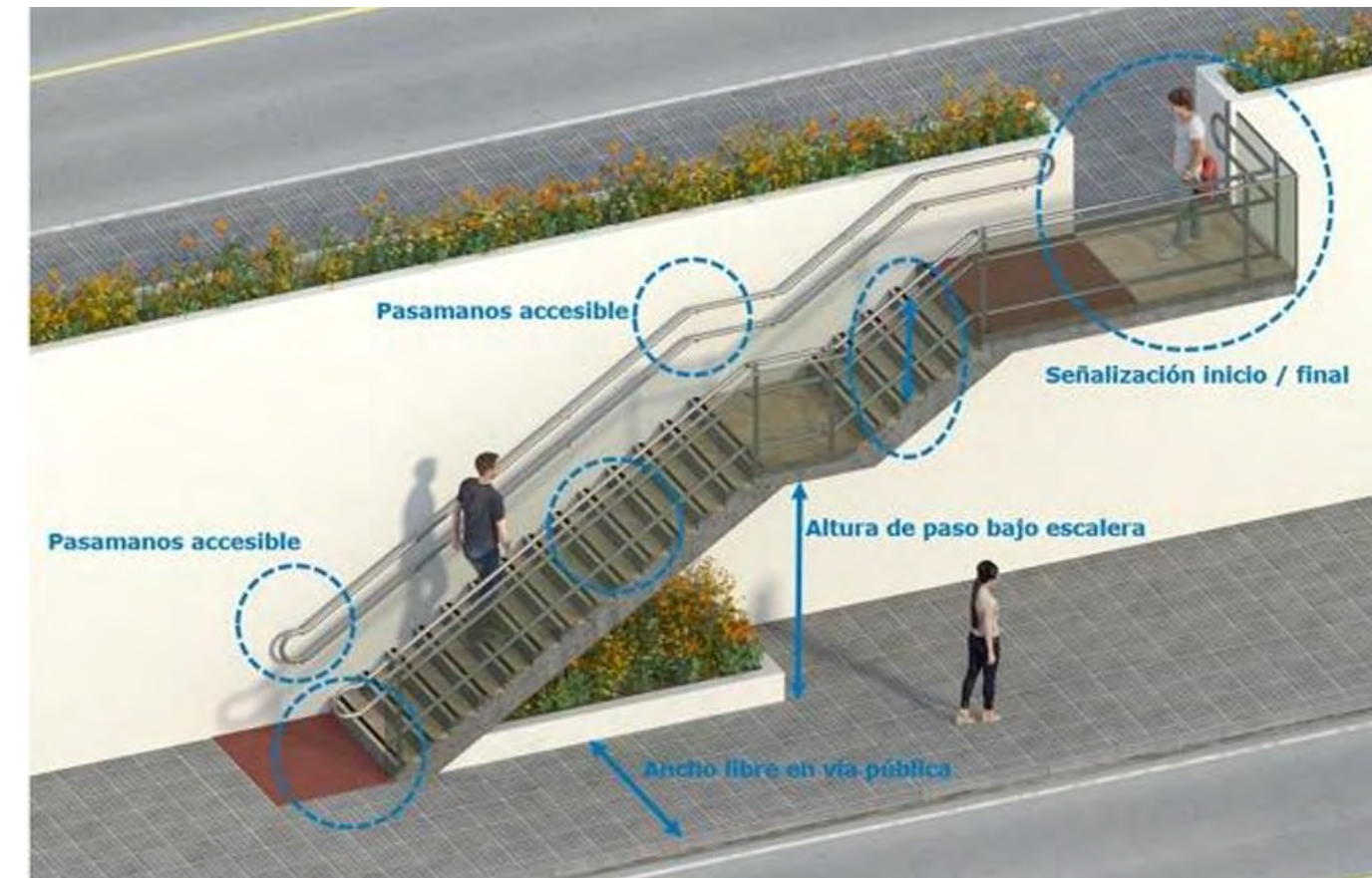
Ilustración 2. Escalera accesible. Fuente: Manual de accesibilidad para espacios públicos urbanizados del Ayuntamiento de Madrid
